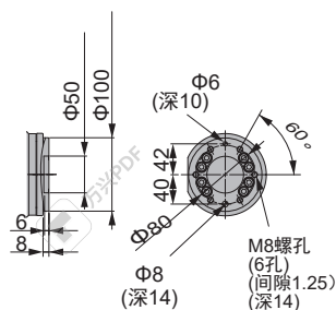
视图 A
